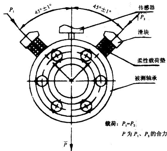
图2 径向载荷装置示意图
