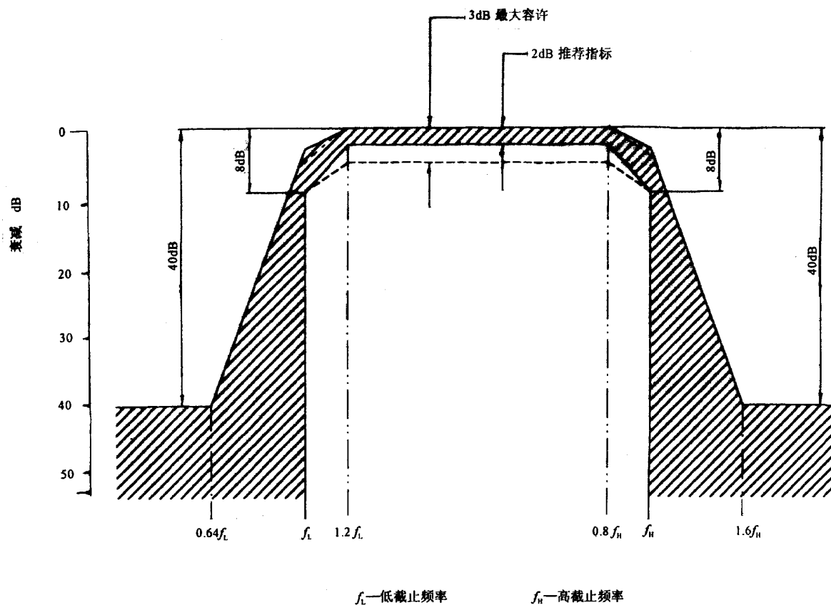
图4 滤波特性
