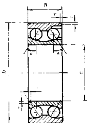
图 1 (有装球缺口的)双列角接触球轴承 00000 型( \alpha=30^\circ )
