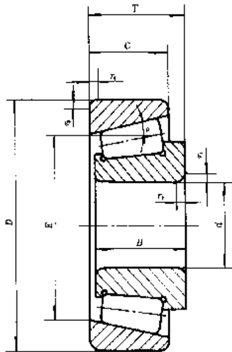
圆锥滚子轴承 30000 型
